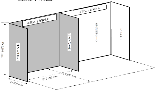
〈基礎小間図〉
