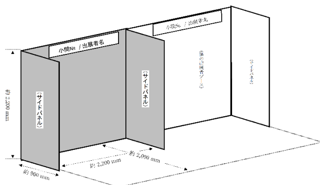
〈基礎小間図〉
